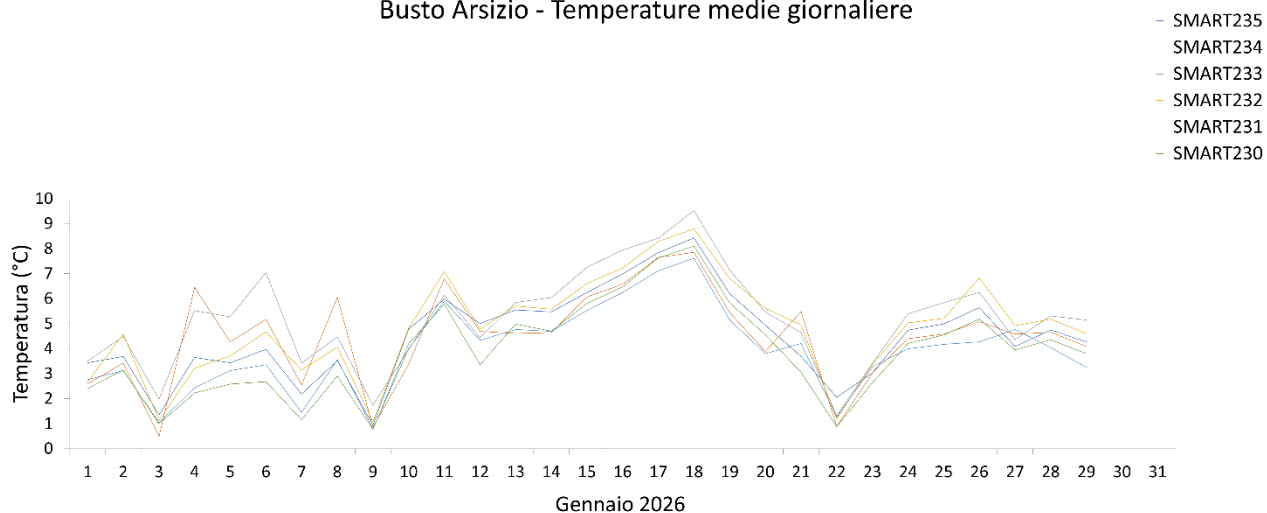
Busto Arsizio - Temperature medie giornaliere
